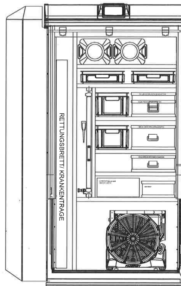
Ausbauvariante 4 für G 1: Zusatzmodul Überdrucklüfter
