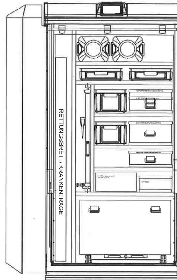
Ausbauvariante 3 für G 1: Zusatzmodul große Aluminiumkiste auf Auszug
