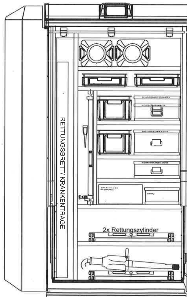
Ausbauvariante 5 für G 1: Zusatzmodul
