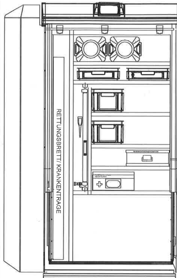
Ausbauvariante 1 für G 1: Ohne Zusatzmodule
